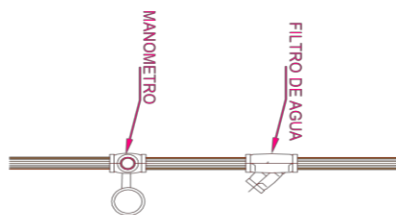
DETALLE MANÓMETRO Y FILTRO
